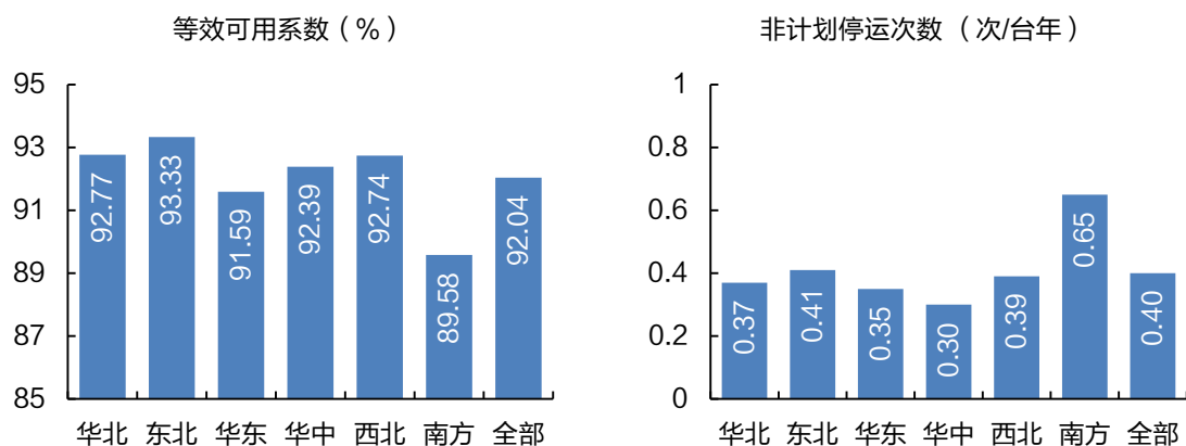
图 1-23 2024 年各地区燃煤机组等效可用系数、非计划停运次数
