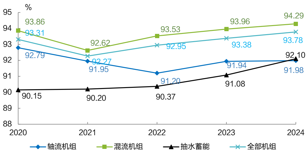
图 1-26 2020-2024 年水电机组等效可用系数
