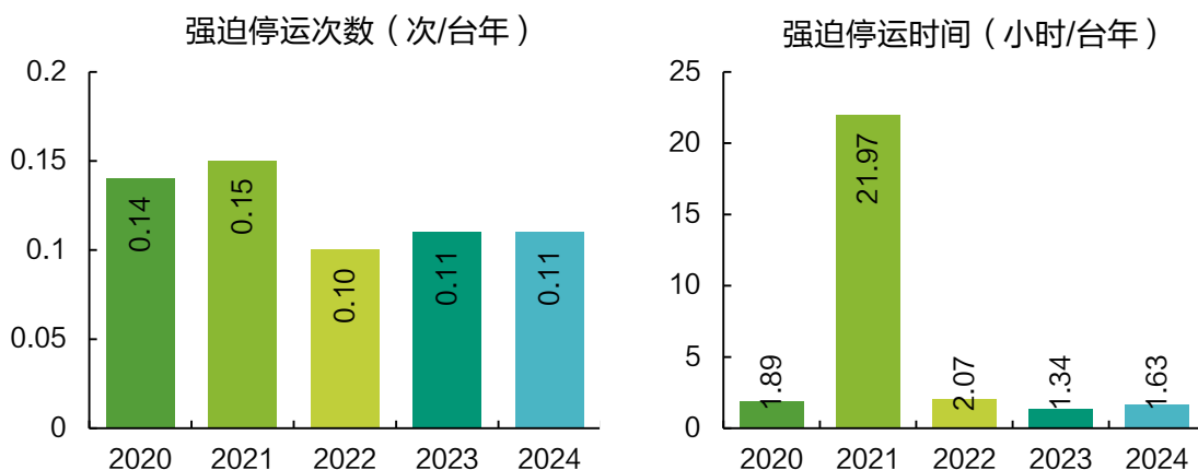
图 1-25 2020-2024 年水电机组强迫停运次数和时间
