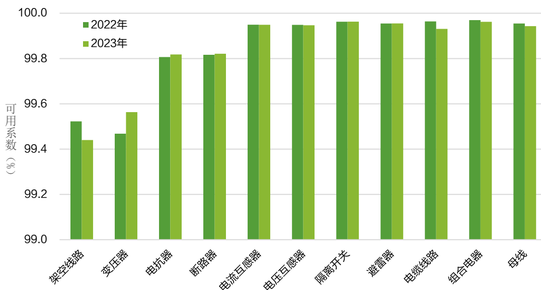
图 3-1 2022、2023 年全国输变电设施可用系数对比
