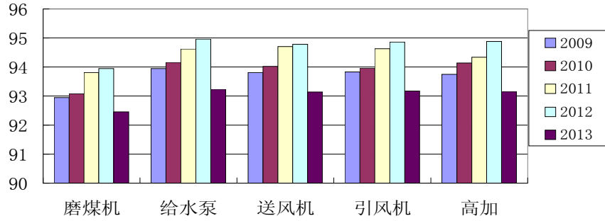
2009—2013 年五种辅助设备的可用系数 %
