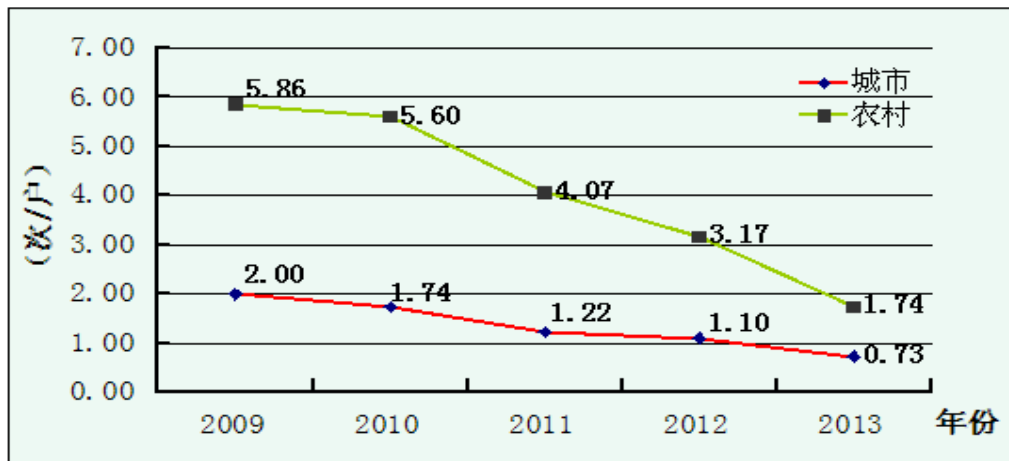
2009-2013 年城市、农村用户平均停电时间趋势
