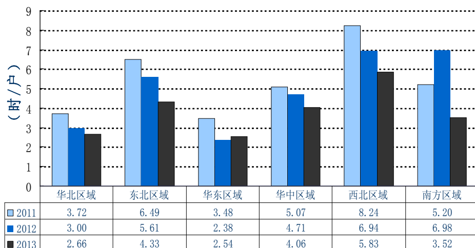
2011-2013 年各区域用户平均停电时间变化趋势（城市）
