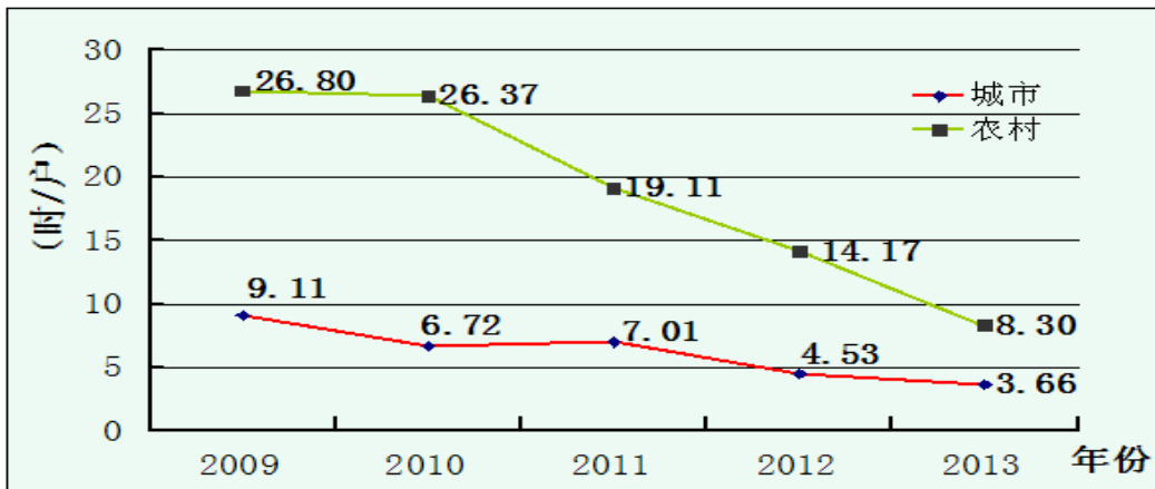
2009-2013 年城市、农村用户平均停电时间趋势
