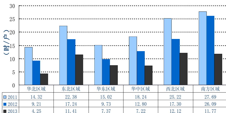
2011-2013 年各区域用户平均停电时间变化趋势（农村）
