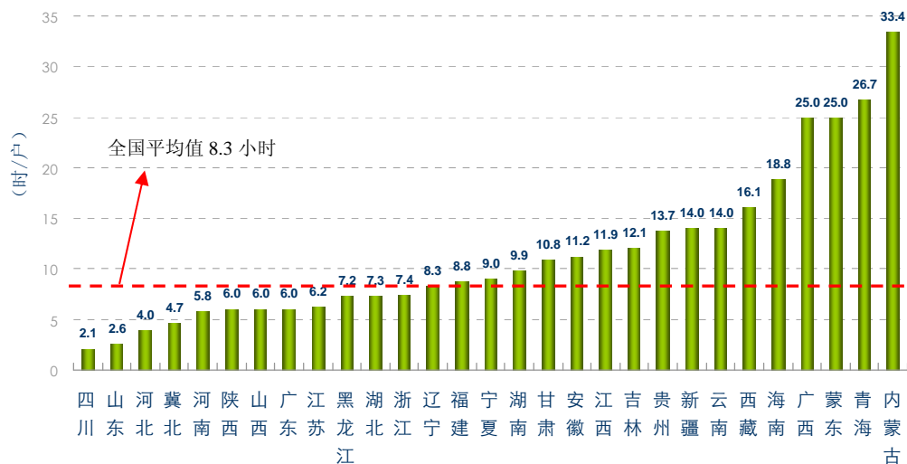
2013 年各省用户平均停电时间分布（农村）
