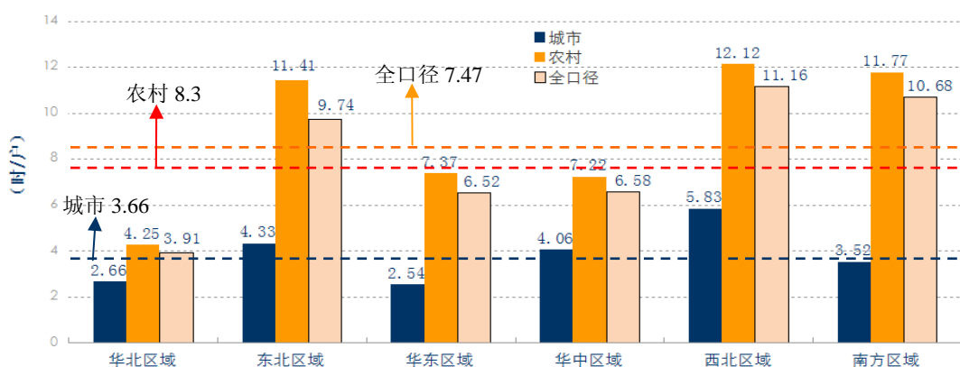
2013 年各区域城市、农村、全口径用户平均停电时间对比
